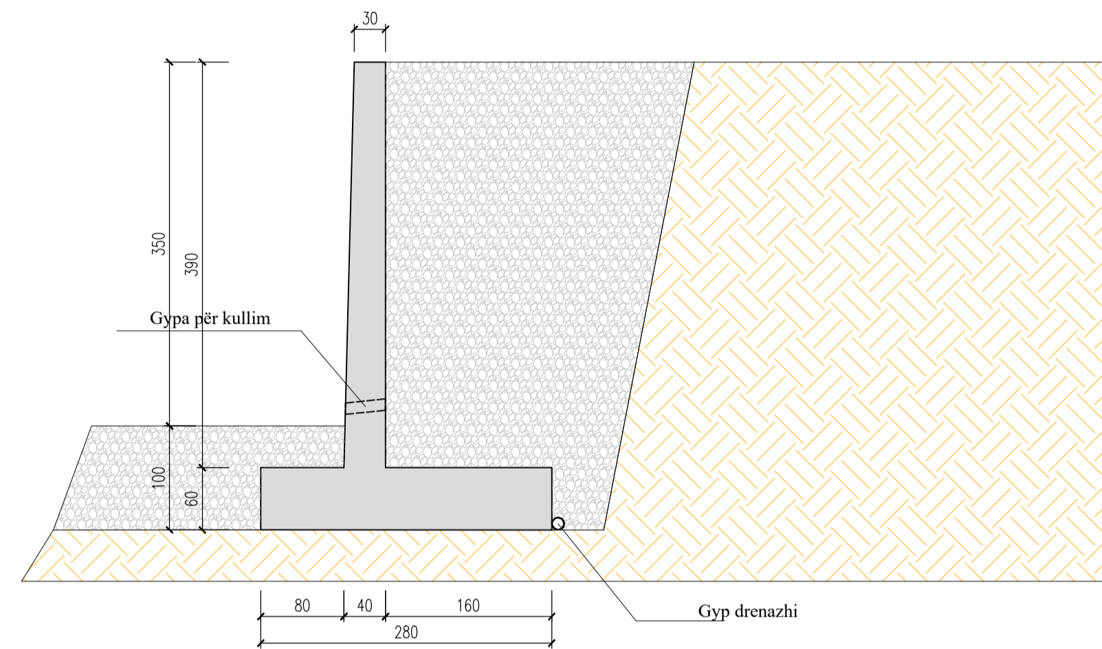
PRERJA TËRTHORE M5(5-5) P:1/50
