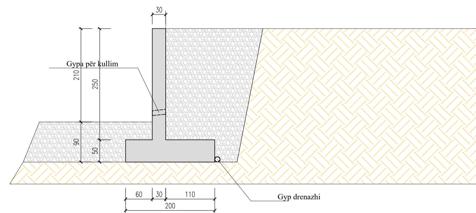
PRERJA TËRTHORE M4(4-4) P:1/50
