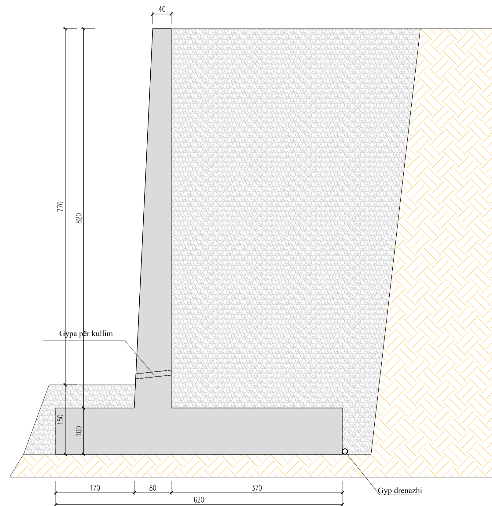
PRERJA TËRTHORE M5(5-5) P:1/50
